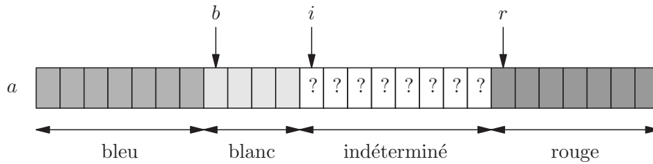
FIG. 5.2 – Le drapeau hollandais
