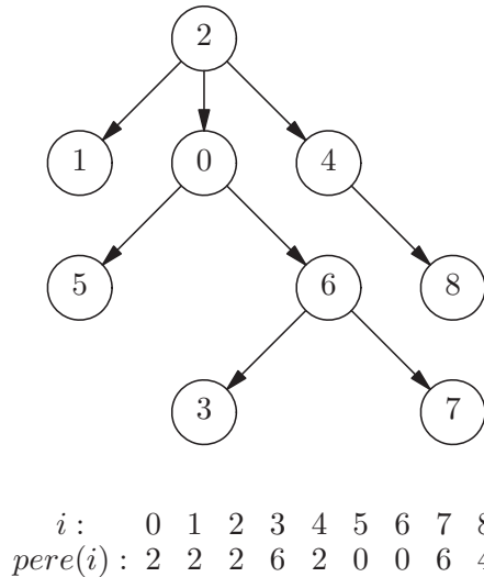
FIG. 1.6 – Une arborescence et son vecteur pere
