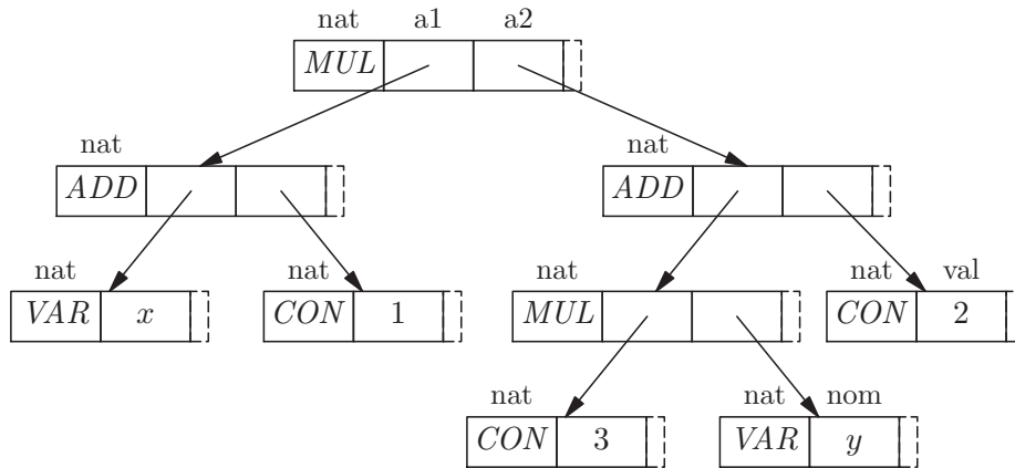
FIG. 2.4 – Représentation d'un arbre de syntaxe abstraite
