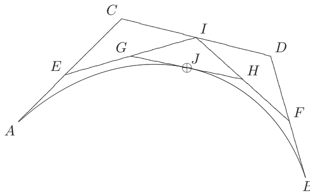
FIG. 8.4 – Décomposition d'une cubique de Bézier
