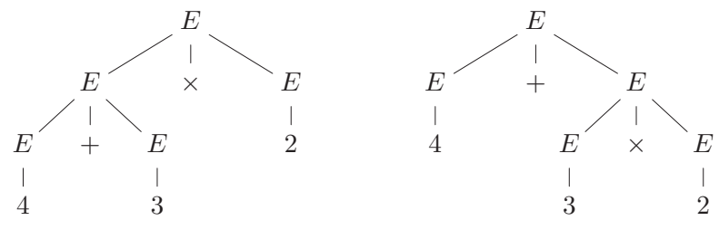
FIG. 2.8 – Grammaire ambiguë
