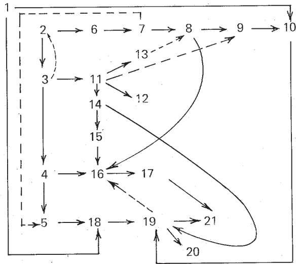
FIG. 1.13 – Un exemple de graphe acyclique
