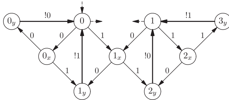
FIG. 7.4 – L'automate d'un additionneur série
