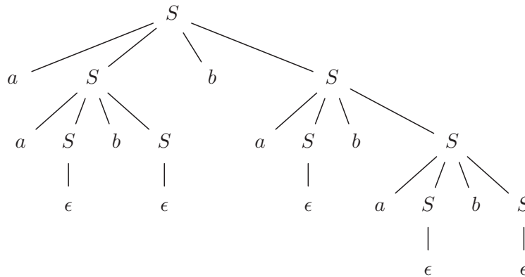
FIG. 2.6 – Arbre de dérivation de aabbabab
