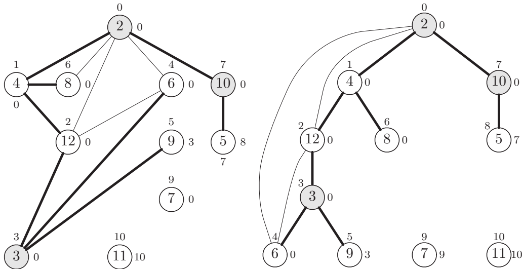
FIG. 1.14 – Points d'articulation dans un graphe non-orienté
