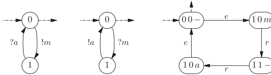
FIG. 7.13 – L'automate d'un simple contrôle de flux sur un réseau. (i) à gauche : l'émetteur ; (ii) au centre : le récepteur ; (iii) à droite : le système en entier
